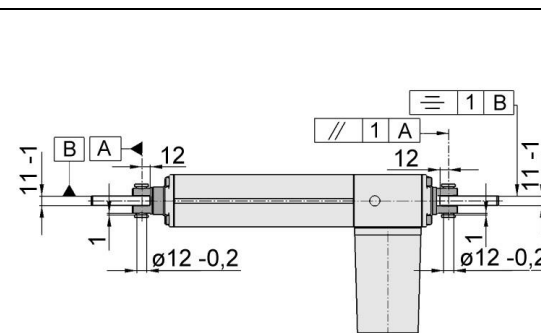
Abb. 6: Ausführung und Abmessungen der Anschlusskonstruktion
