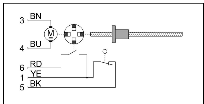
Abb. 3: Schaltbild und Belegung für Wegmesssystem
