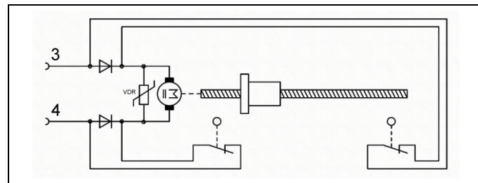
Fig. 12: Modulo di sollevamento Standard (8918-0X-X0-E)
