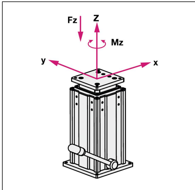
Fig. 5: Forze trasversali
