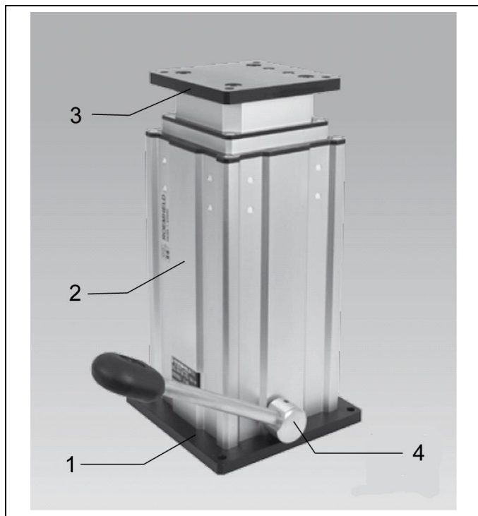
Fig. 2: Componenti
