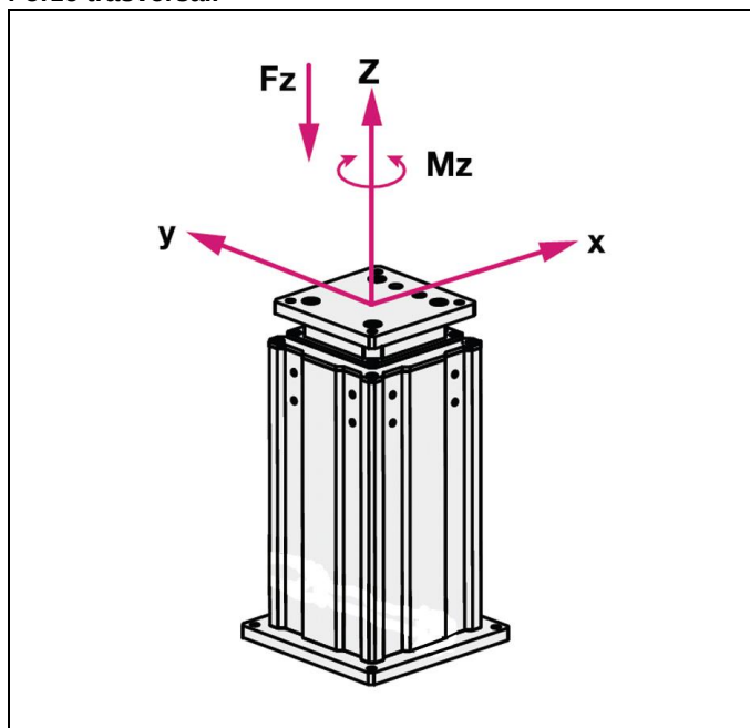
Fig. 11: Forze trasversali
