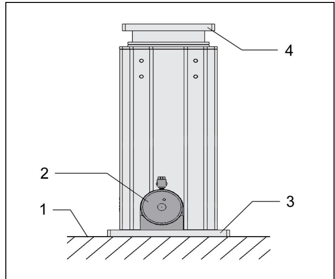
Fig. 8: Principe de la fixation
