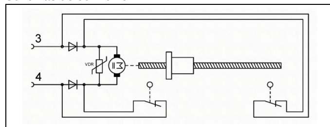
Fig. 12: Module de levage standard (8918-0X-X0-E)
